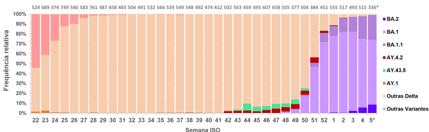
Figura 2. Evolução da frequência relativa semanal das (sub)-linhagens de SARS-CoV-2 em circulação em Portugal entre as semanas ISO 22 (31 de maio a 6 de junho, 2021) e 5 (31 de janeiro a 6 de fevereiro de 2022). Os valores acima de cada barra indicam o número de sequências avaliadas por semana no âmbito das amostragens aleatórias nacionais. O gráfico destaca: i) as (sub)linhagens BA.1, BA.1.1 e BA.2 (classificadas como Omicron pela OMS) e ii) outras sub-linhagens Delta de interesse (AY.1, AY.4.2 e AY.43.5). *É de esperar a existência de algumas flutuações nas frequências apresentadas para a última semana em análise (semana ISO 5), na medida em que ainda estão a ser apurados dados relativos a esse período.
