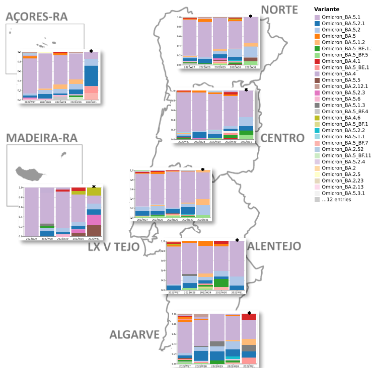
Figura 2: Evolução da frequência relativa semanal das (sub)-linhagens de SARS-CoV-2 em circulação em Portugal por Região de Saúde, entre as semanas ISO 27 (04/07/22 a 10/07/22) e 31 (01/08/22 a 07/08/22). É de esperar a existência de algumas flutuações nas frequências apresentadas para a última semana em análise (semana ISO 31*), na medida em que ainda estão a ser apurados dados relativos a esse período. Consulte no website este, e outros, gráficos de forma interativa.
