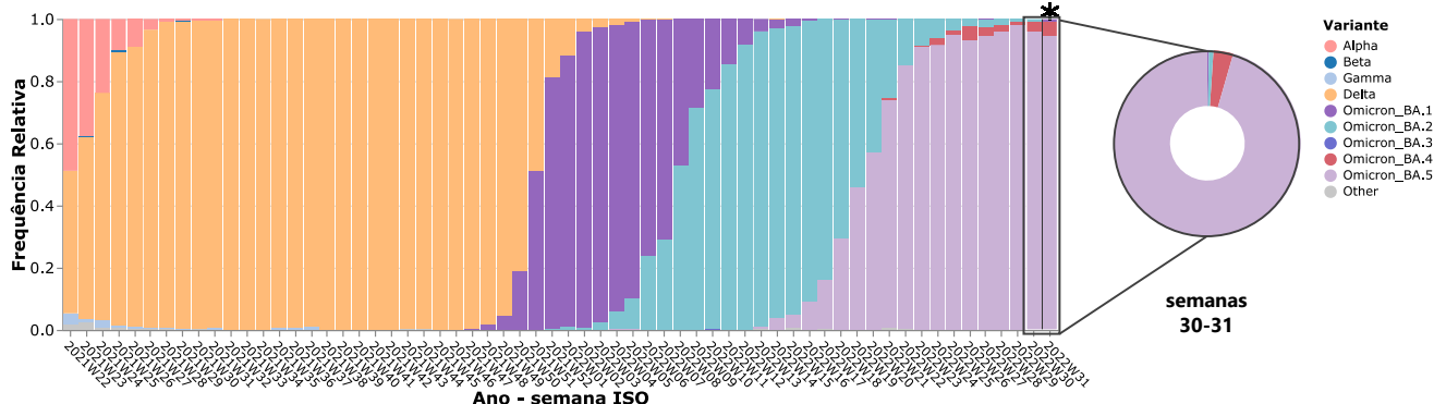
Figura 1: Evolução da frequência relativa semanal das variantes de SARS-CoV-2 em circulação em Portugal entre as semanas ISO 22 (31/05/21 a 06/06/21) e 31 (01/08/22 a 07/08/22). É de esperar a existência de algumas flutuações nas frequências apresentadas para a última semana em análise (semana ISO 31*), na medida em que ainda estão a ser apurados dados relativos a esse período. Consulte no website este, e outros, gráficos de forma interativa.
