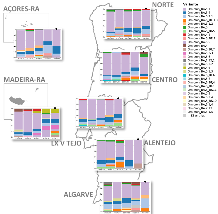
Figura 2: Evolução da frequência relativa semanal das (sub)-linhagens de SARS-CoV-2 em circulação em Portugal por Região de Saúde, entre as semanas ISO 28 (11/07/22 a 17/07/22) e 32 (08/08/22 a 14/08/22). É de esperar a existência de algumas flutuações nas frequências apresentadas para a última semana em análise (semana ISO 32*), na medida em que ainda estão a ser apurados dados relativos a esse período. Consulte no website este, e outros, gráficos de forma interativa.
