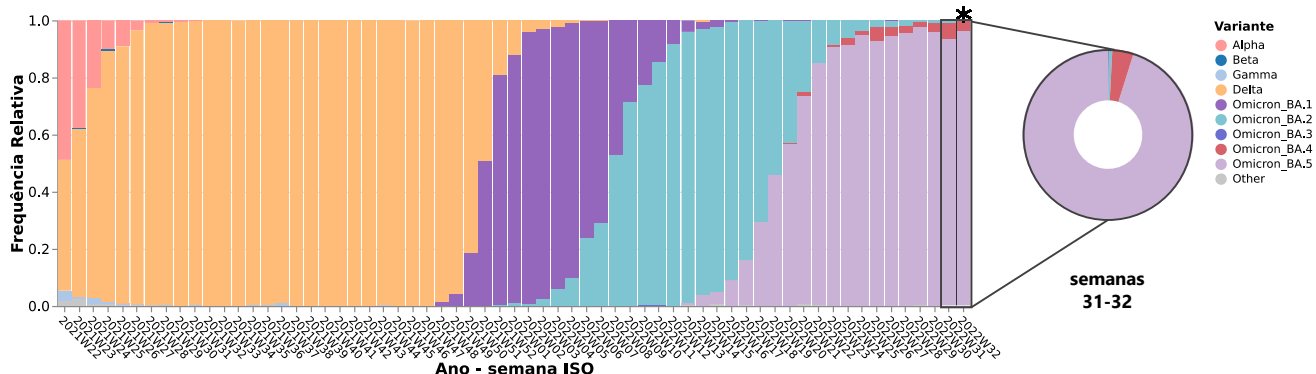
Figura 1: Evolução da frequência relativa semanal das variantes de SARS-CoV-2 em circulação em Portugal entre as semanas ISO 22 (31/05/21 a 06/06/21) e 32 (08/08/22 a 14/08/22). É de esperar a existência de algumas flutuações nas frequências apresentadas para a última semana em análise (semana ISO 32*), na medida em que ainda estão a ser apurados dados relativos a esse período. Consulte no website este, e outros, gráficos de forma interativa.
