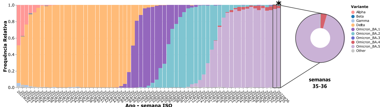
Figura 1: Evolução da frequência relativa semanal das variantes de SARS-CoV-2 em circulação em Portugal entre as semanas ISO 22 (31/05/21 a 06/06/21) e 36 (05/09/22 a 11/09/22). É de esperar a existência de algumas flutuações nas frequências apresentadas para a última semana em análise (semana ISO 36*), na medida em que ainda estão a ser apurados dados relativos a esse período. Consulte no website este, e outros, gráficos de forma interativa.
