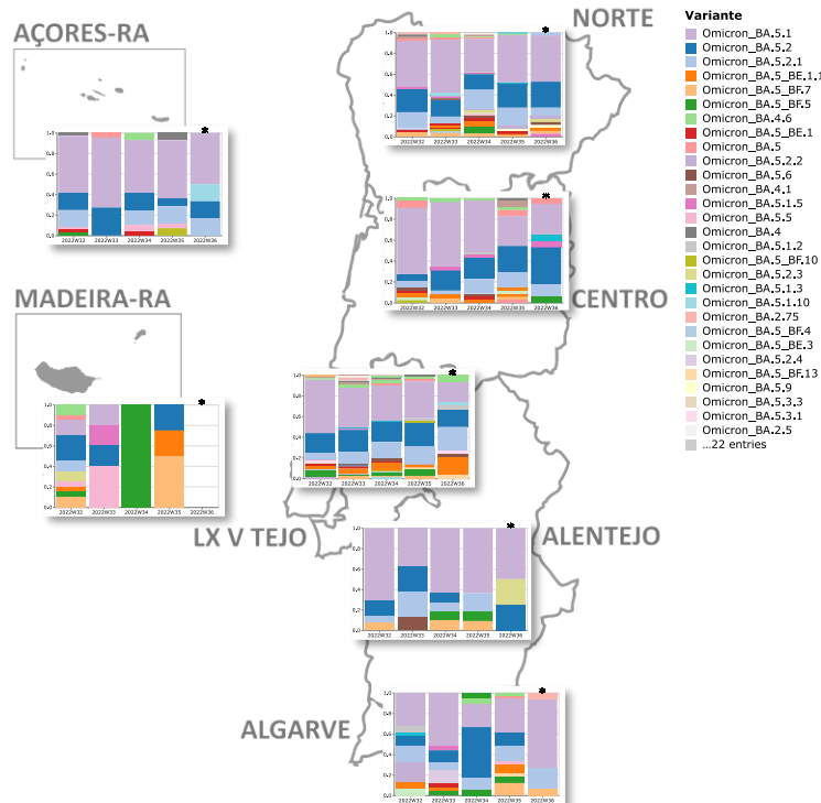
Figura 2: Evolução da frequência relativa semanal das (sub-)linhagens de SARS-CoV-2 em circulação em Portugal por Região de Saúde, entre as semanas ISO 32 (08/08/22 a 14/08/22) e 36 (05/09/22 a 11/09/22). A frequência relativa a nível regional deve ser interpretada com cautela devido aos números reduzidos de amostras em algumas regiões. É de esperar a existência de algumas flutuações nas frequências apresentadas para a última semana em análise (semana ISO 36*), na medida em que ainda estão a ser apurados dados relativos a esse período. Consulte no website este, e outros, gráficos de forma interativa.
