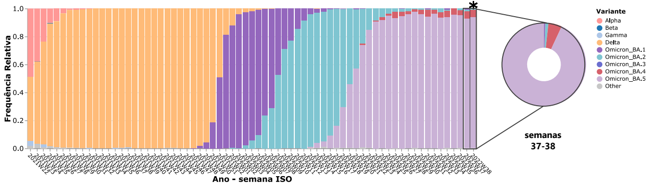
Figura 1: Evolução da frequência relativa semanal das variantes de SARS-CoV-2 em circulação em Portugal entre as semanas ISO 22 (31/05/21 a 06/06/21) e 38 (19/09/22 a 25/09/22). É de esperar a existência de algumas flutuações nas frequências apresentadas para a última semana em análise (semana ISO 38*), na medida em que ainda estão a ser apurados dados relativos a esse período. Consulte no website este, e outros, gráficos de forma interativa.
