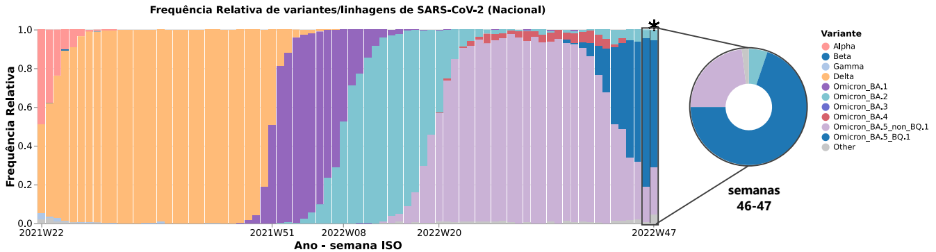
Figura 1: Evolução da frequência relativa semanal das variantes de SARS-CoV-2 em circulação em Portugal entre as semanas ISO 22 (31/05/21 a 06/06/21) e 47 (21/11/22 a 27/11/22). É de esperar a existência de algumas flutuações nas frequências apresentadas para a última semana em análise (semana ISO 47*), na medida em que ainda estão a ser apurados dados relativos a esse período. Consulte no website este e outros gráficos de forma interativa.
