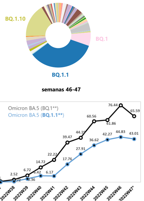
Figura 2: Evolução da frequência relativa da sub-linhagem BQ.1 e suas descendentes BQ.1.1 em Portugal. O gráfico circular mostra a distribuição da frequência relativa de sub-linhagens de SARS-CoV-2 no período das semanas 46 e 47 (entre 14 e 27 de novembro de 2022), destacando as sub-linhagens que representam mais de 5% das sequências analisadas neste período . A evolução de BQ.1** e BQ.1.1** nas últimas 11 semanas é ilustrada no gráfico de linhas. É de esperar a existência de algumas flutuações nas frequências apresentadas para a última semana em análise (semana ISO 47*), na medida em que ainda estão a ser apurados dados relativos a esse período. **as frequências apresentadas são relativas às sub-linhagens e suas descendentes. Consulte no website outros gráficos de forma interativa.
